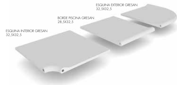
SISTEMA PISCINA GRESAN / GRESAN SYSTEM POOL / SYSTÈME PISCINE GRESAN
