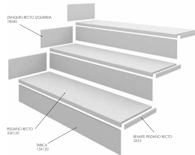
SISTEMA PELDAÑO RECTO / PELDAÑO RECTO SYSTEM / SYTÈME PELDAÑO RECTO
