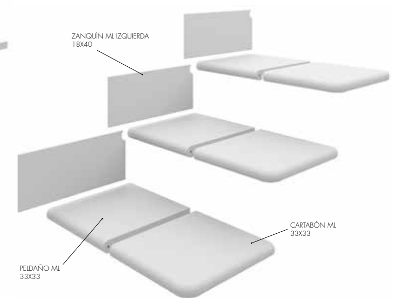
SISTEMA PELDAÑO FIORENTINO / PELDAÑO FIORENTINO SYSTEM / SYSTÈME PELDAÑO FIORENTINO
