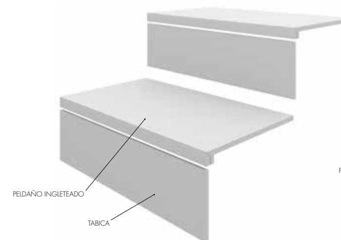
SISTEMA PELDAÑO INGLETEADO / PELDAÑO INGLETEADO SYSTEM / SYSTÈME PELDAÑO INGLETEADO
