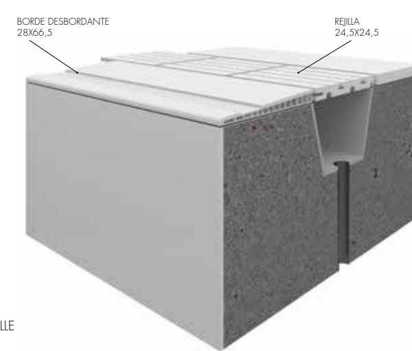
SISTEMA BORDE DESBORDANTE / OVERFLOW / À DÉPORDMENT
